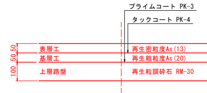
施工要領図
